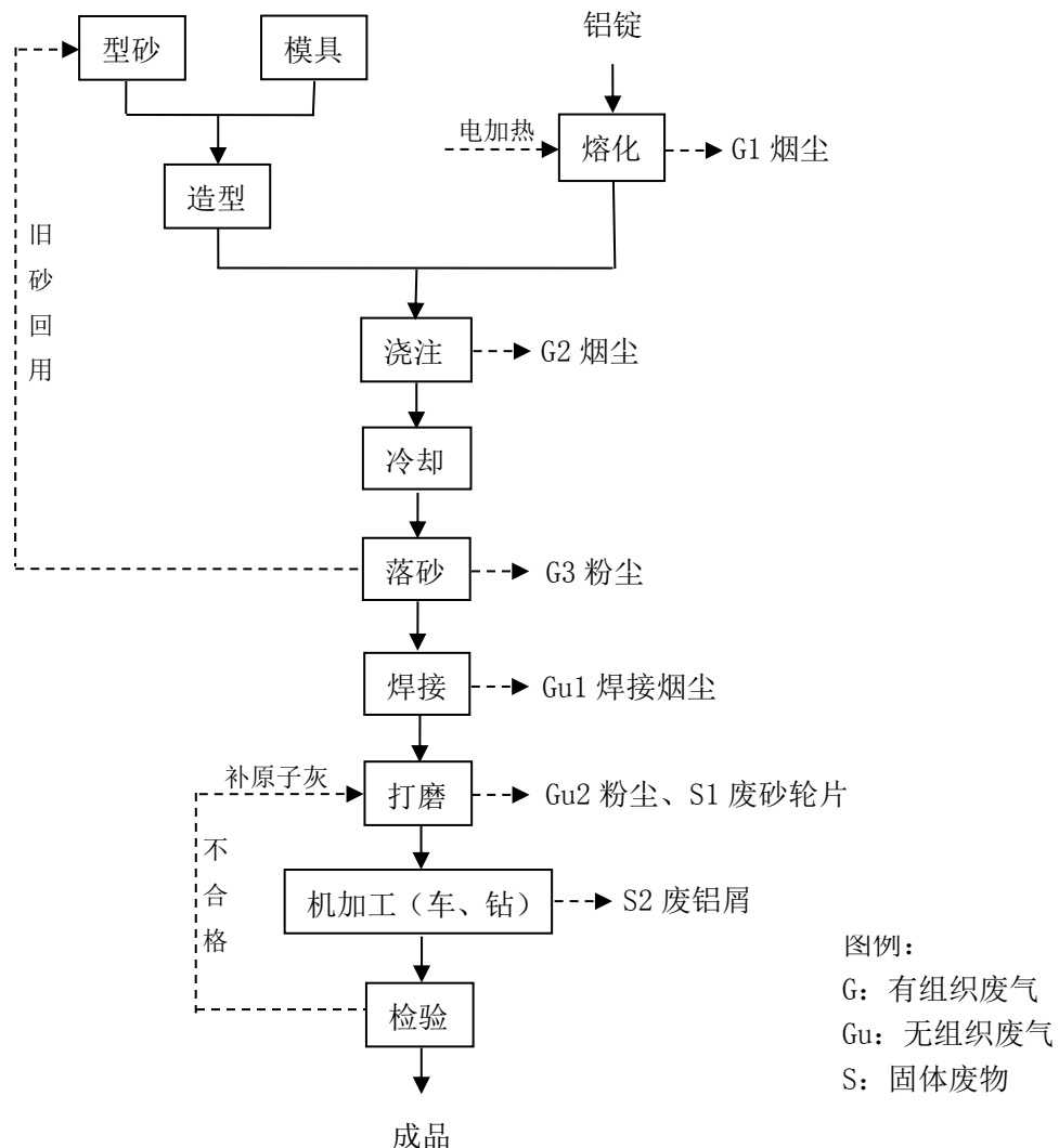
图 1 照明灯具工艺流程图
