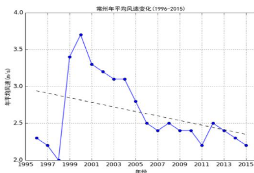
图2 常州 (1996-2015年) 年平均风速 (单位: m/s, 虚线为趋势线)
