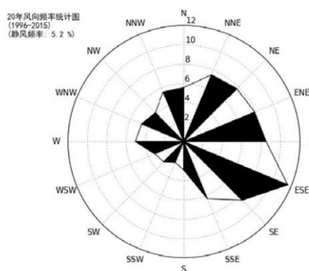
图1 常州风向玫瑰图 (静风频率5.2%)
